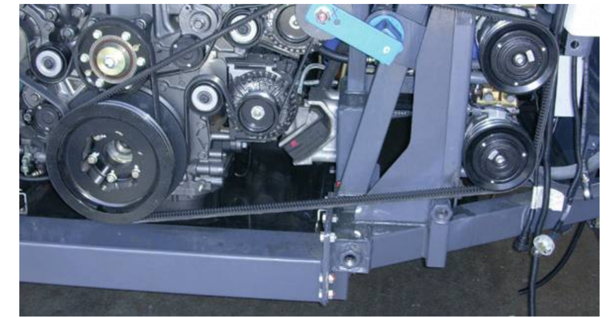
Compresor de refrigeración diseñado con ROSTA ESL ®.
